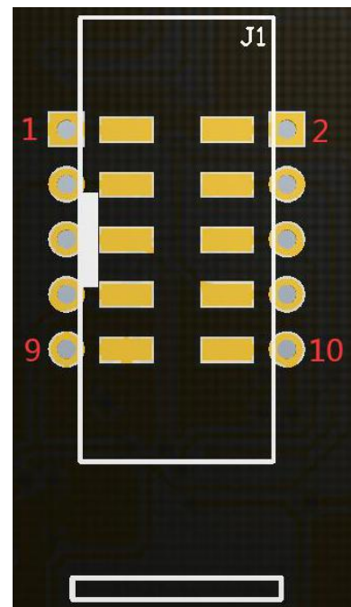
B. 2.54mm 2*5P 牛角座
