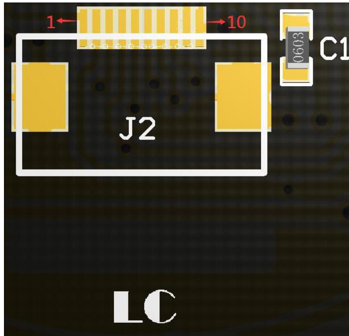
A. 0.5mm 10P FPC 座
